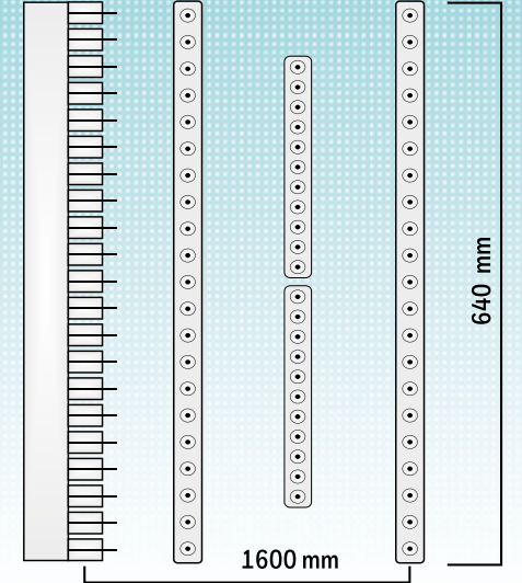
4X21 ÇOKLU DELİK MAKİNASI 4X21 MULTI BORING MACHINE
