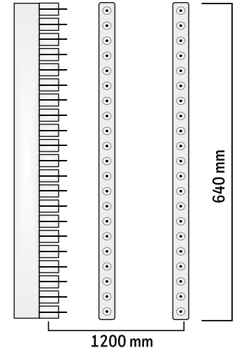
3X21 ÇOKLU DELİK MAKİNASI 3X21 MULTI BORING MACHINE
